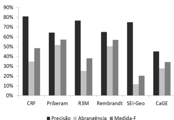
Figura 2: Desempenho do NERP-CRF comparado graficamente com os sistemas no ‘Teste 2’.
