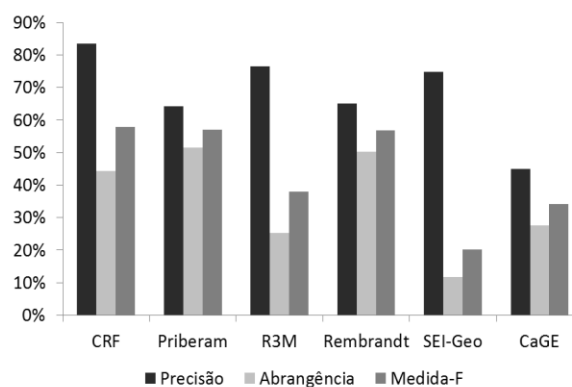
Figura 1: Desempenho do NERP-CRF comparado graficamente com os sistemas no ‘Teste 1’.
