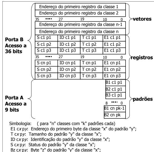
Figura 4 - Organização interna das DPRAMs.
