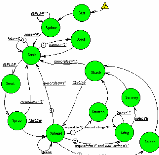
Figura 6 - Máquina de estados de controle das pico-CPU's.
