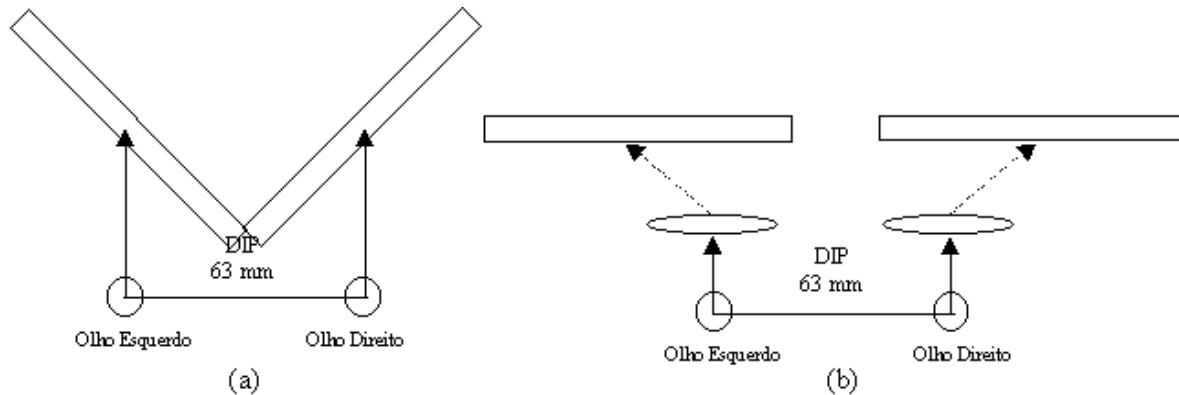
Figura 3.8 – Posicionamento dos alternativo monitores em relação aos olhos
