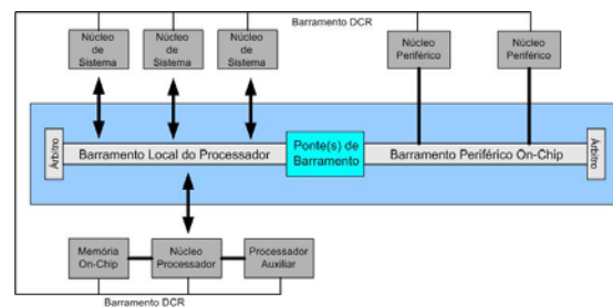
Figura 3 - Arquitetura de barramento CoreConnect .
