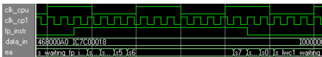
Figura 25 - Instrução de ponto flutuante de latência de 12 ciclos de relógios sendo executada em uma relação de frequência CP1/CPU = 8.
